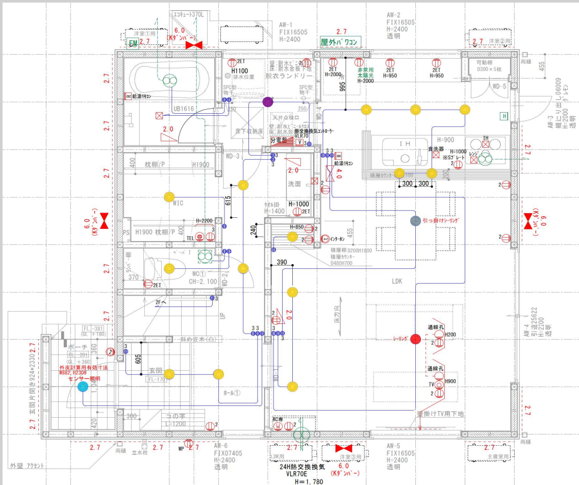
1階
